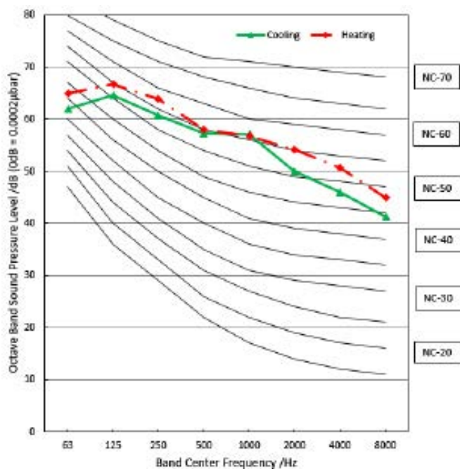
KUE-125 DVR13
