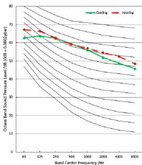
KUE-125 DVR13
