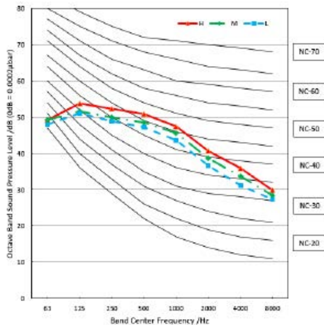
KPD-125 DR13
