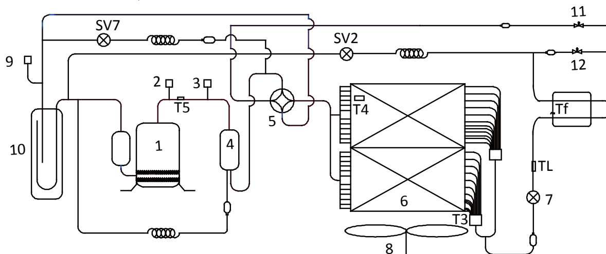
Illustration 2-4.1 : Schéma de la tuyauterie 7/8/9/10 CV
