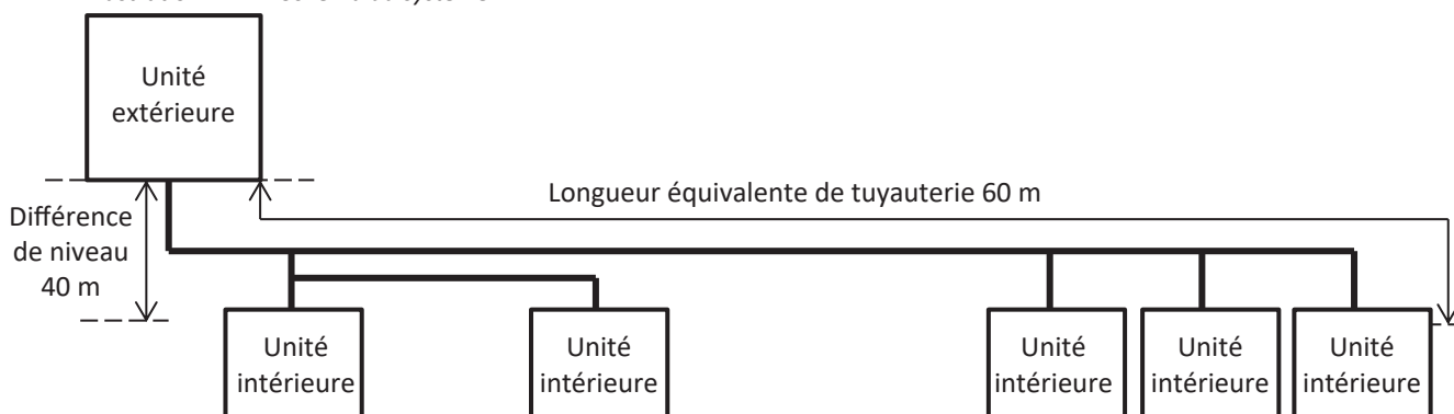
Illustration 1-4.2 : Schéma du système
