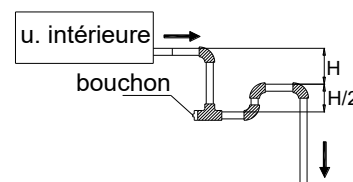
Illustration 3-5.6 : Pièges à eau de la tuyauterie d'évacuation
