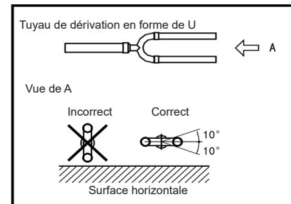
Illustration 3-4.8 : Orientation des raccords de dérivation
