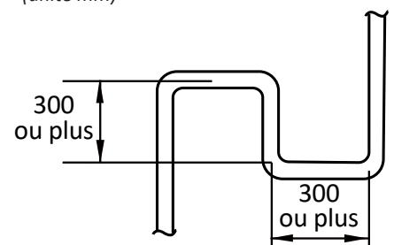
Illustration 3-3.1 : Retour d'huile courbé (unité mm)
