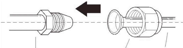
Tubo interior de la unidad Tuerca abocinada Tubo Fig. 6.7
