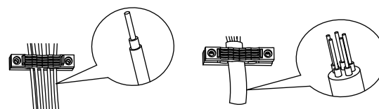
Metoda 1 de prindere cu clemă
