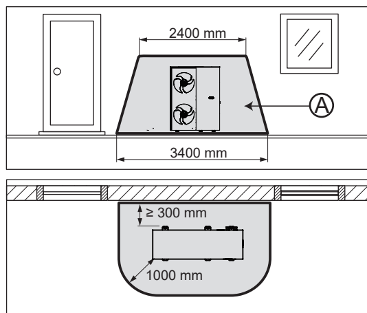
Aufstellen des Außengeräts vor einer Außenwand
