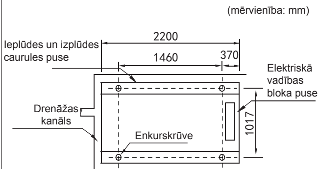
6-6. attēls. 110 KW modeļa uzstādīšanas izmēru principshēma, skats no augšas
