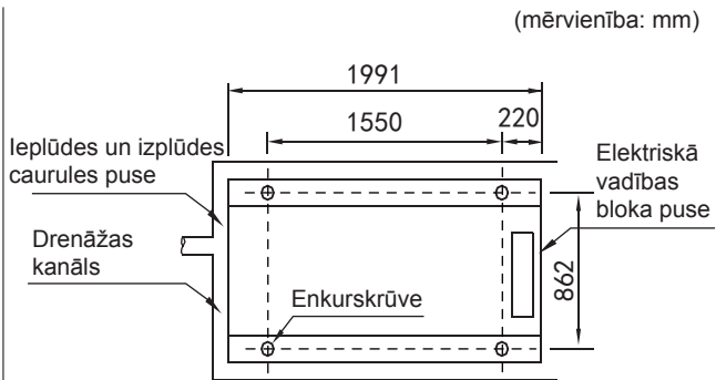
6-5. attēls. 65 KW modeļa uzstādīšanas izmēru principshēma, skats no augšas
