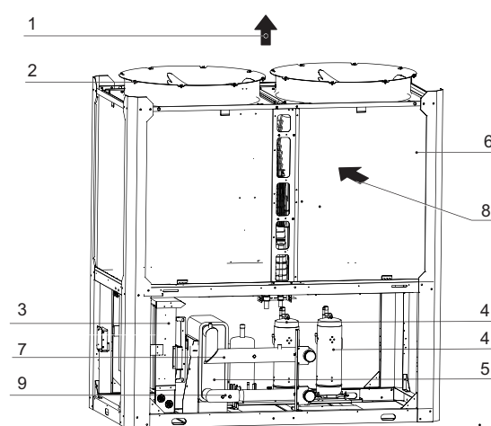
8-2. attēls. 110 KW modeļa galvenās daļas
