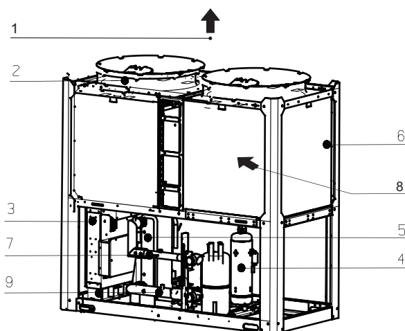
8-1. attēls. 65 KW modeļa galvenās daļas
