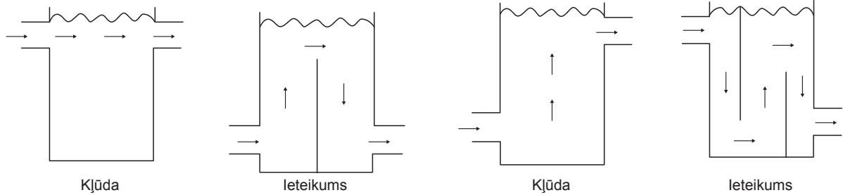
8-20. attēls. Rezerves tvertnes konstrukcija
