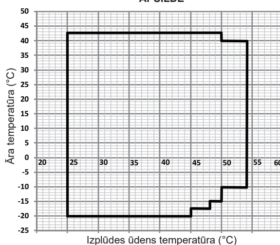
1-1-2. attēls. Apsildes darba diapazons
