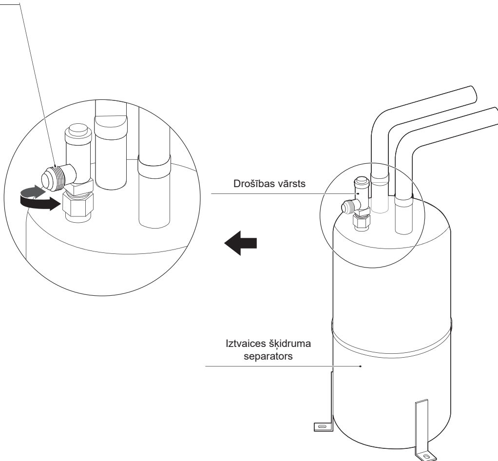
11-1. attēls. Drošības vārsta nomaiņa
