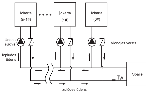
8-34. attēls. Vairāku ūdens sūkņu uzstādīšana
