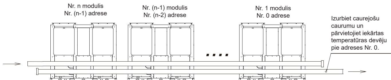
8-32. attēls. Vairāku moduļu uzstādīšana (ne vairāk kā 8 moduļi), modelim KEM-180 DRS5 KH
