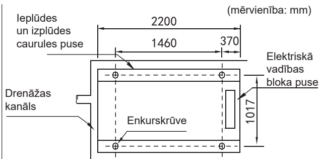
6-7. attēls. Modeļu KEM-90 DRS5 KH un MC-SU140M-RN8L-B uzstādīšanas izmēru principshēma, skats no augšas
