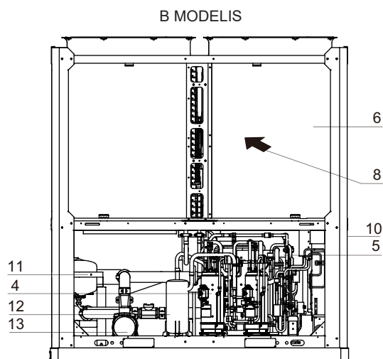
8-4. attēls. Modeļa KEM-180 DRS5 KH galvenās daļas (Attēls sniegts, tikai lai parādītu galveno daļu aptuvenu izvietojumu.)
