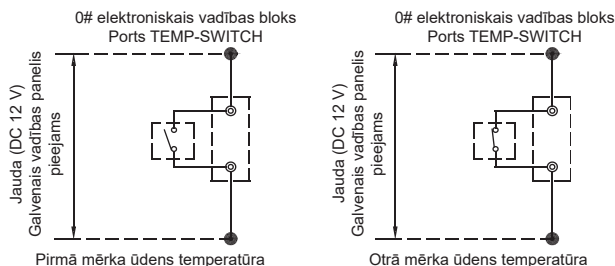
8-22. attēls. Temperatūras pārslēgšanas vājstrāvas elektriskā porta elektroinstalācija
