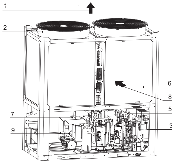
8-2. attēls. Modeļa MC SU90M-RN8L-B galvenās daļas (Attēls sniegts, tikai lai parādītu galveno daļu aptuvenu izvietojumu.)
