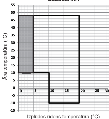
1-1-1. attēls. Dzesēšanas darba diapazons
