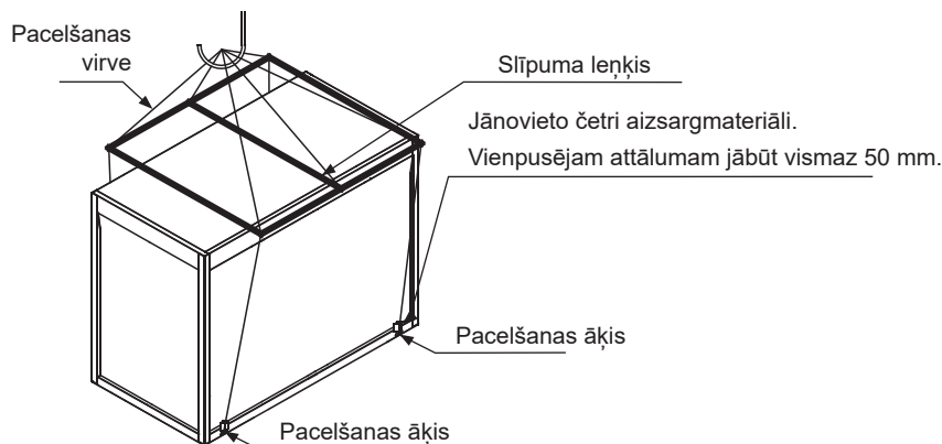
3-1. attēls. Iekārtas pacelšana
