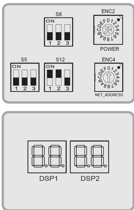
8-14. attēls. Displeja opcijas
