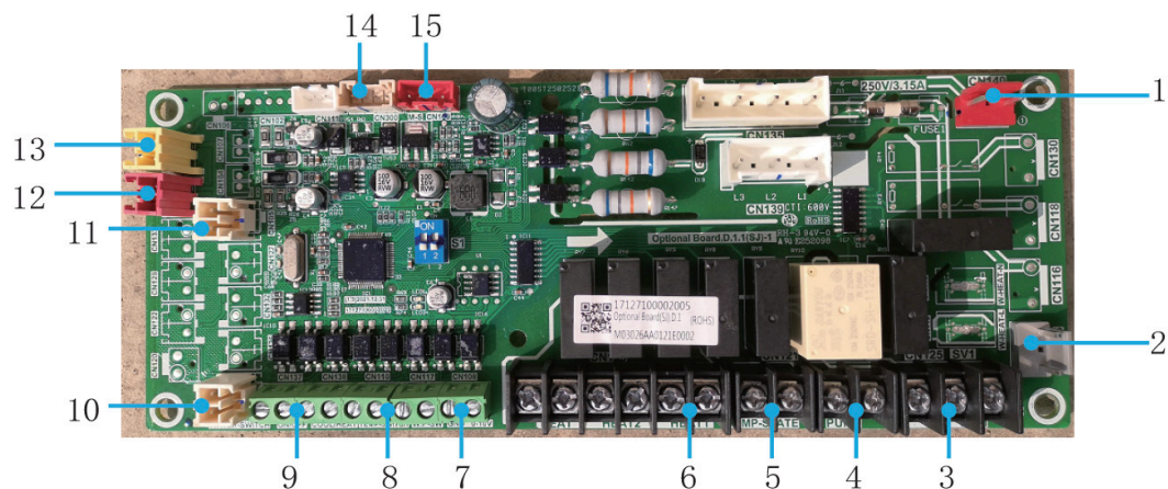
8-10. attēls. Modeļu MC-SU75-RN8L-B un MC-SU140-RN8L-B saistītais vadības panelis
