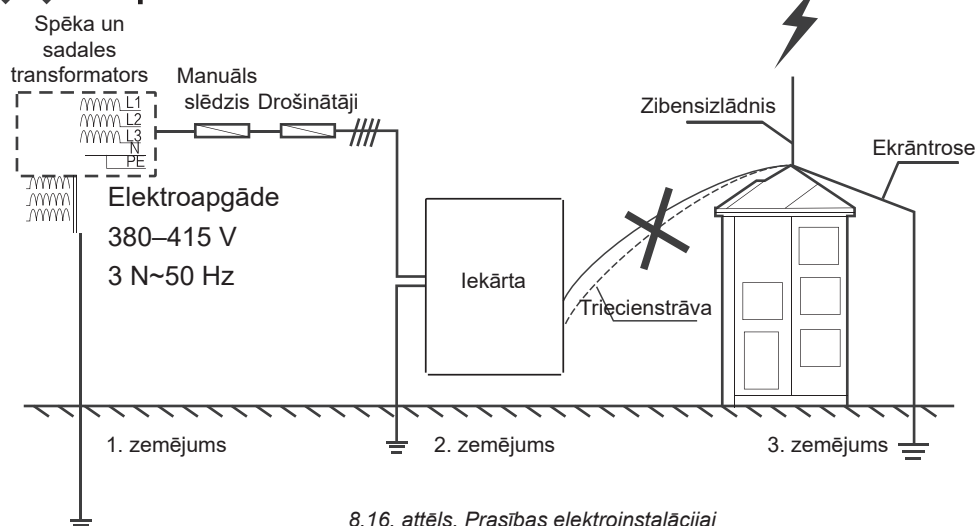
8.16. attēls. Prasības elektroinstalācijai
