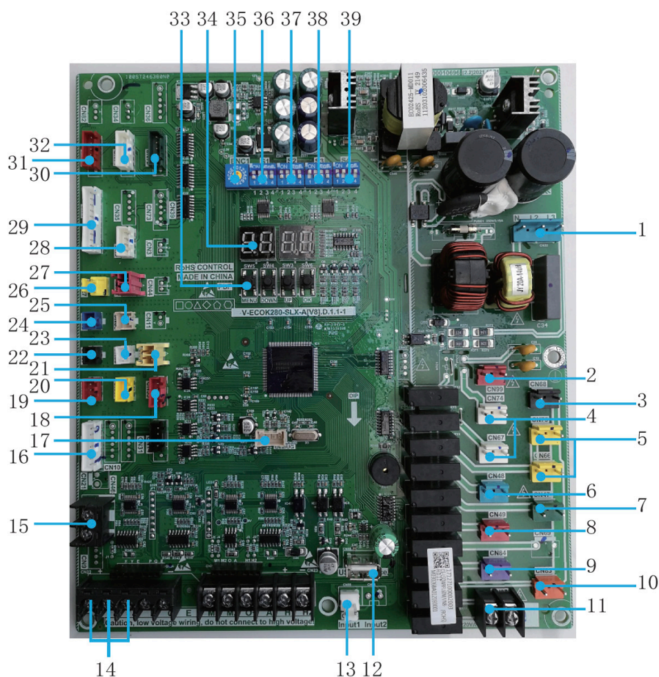
8-9. attēls. Modeļu KEM-75 DRS5 KH un KEM-140 DRS5 KH galvenais panelis
