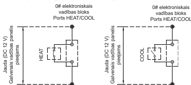
8-21-2. attēls. Apsildes/dzesēšanas vājstrāvas elektriskā porta elektroinstalācija
