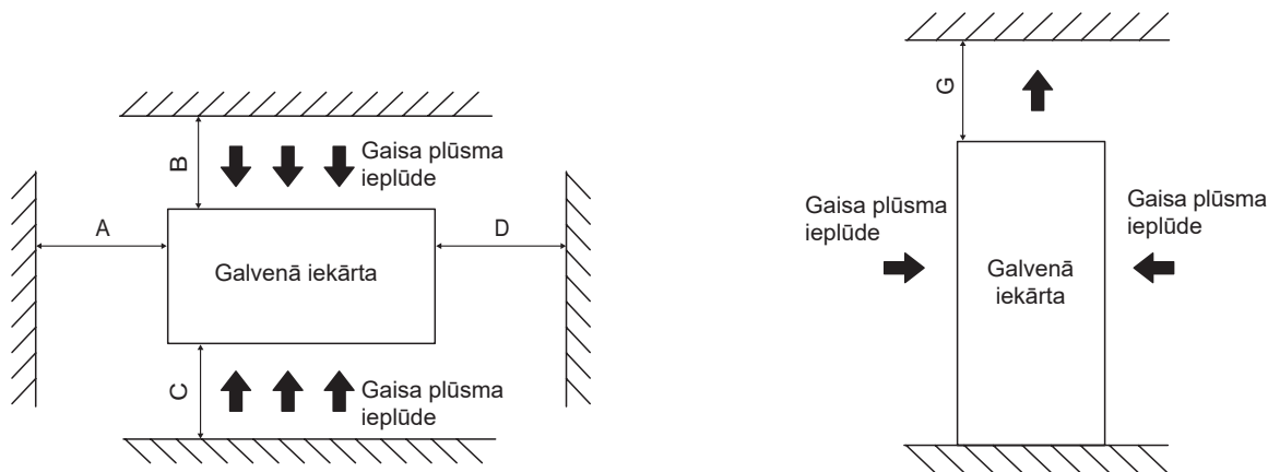
6-3. attēls. Vienas iekārtas uzstādīšana
