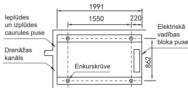
6-6. attēls. Modeļa KEM-75 DRS5 KH uzstādīšanas izmēru principshēma, skats no augšas
