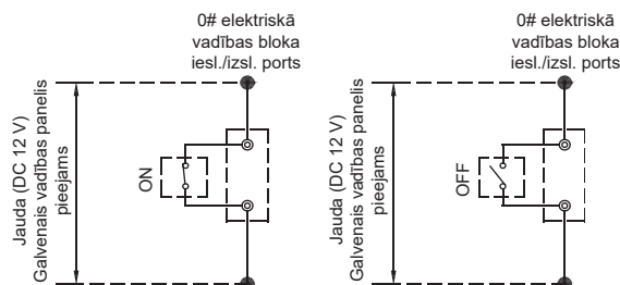
8-21-1. Ieslēgšanas/izslēgšanas vājstrāvas elektrisko portu elektroinstalācija
