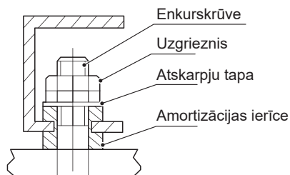
6-9. attēls. Trokšņu slāpētāja uzstādīšana
