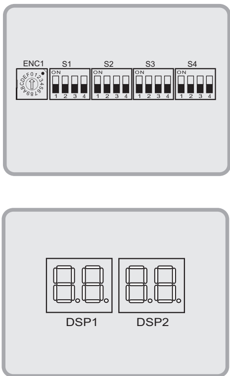
8-13. attēls. Displeja opcijas
