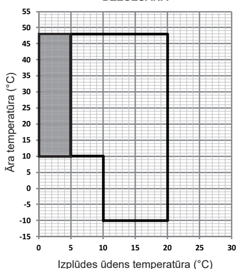
1-2-1. attēls. Dzesēšanas darba diapazons
