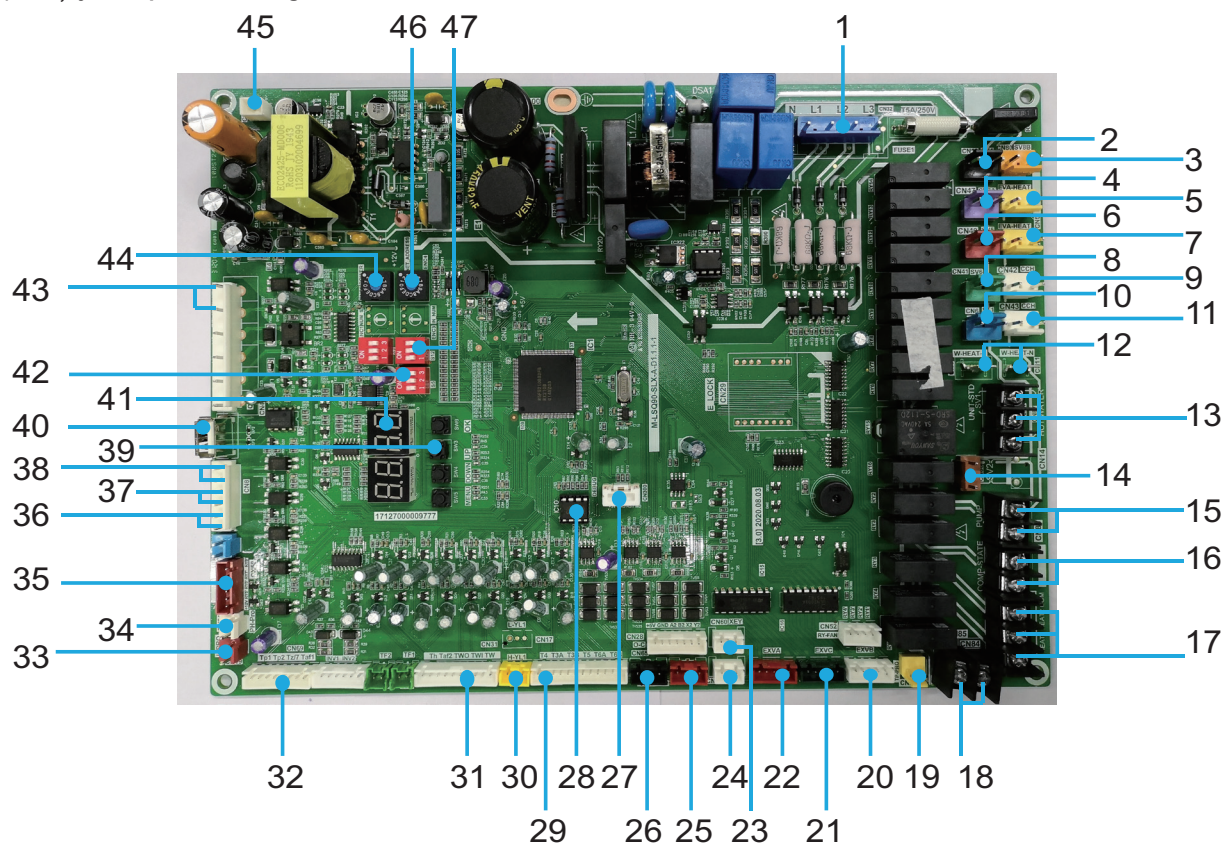
8-11. attēls. Modeļu KEM-90 DRS5 KH un KEM-180 DRS5 KH galvenais PCB
