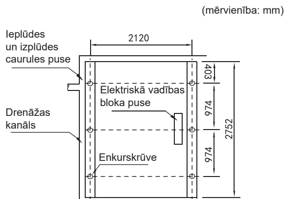
6-8. attēls. Modeļa KEM-180 DRS5 KH uzstādīšanas izmēru principshēma, skats no augšas
