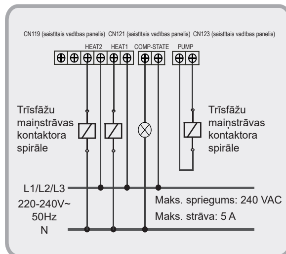
8-19. attēls. Ūdens sūkņa, cauruļu papildu sildītāja un kompresora stāvokļa maiņstrāvas indikatora elektroinstalācija (tikai modeļiem KEM-75 DRS5 KH un KEM-140 DRS5 KH)
