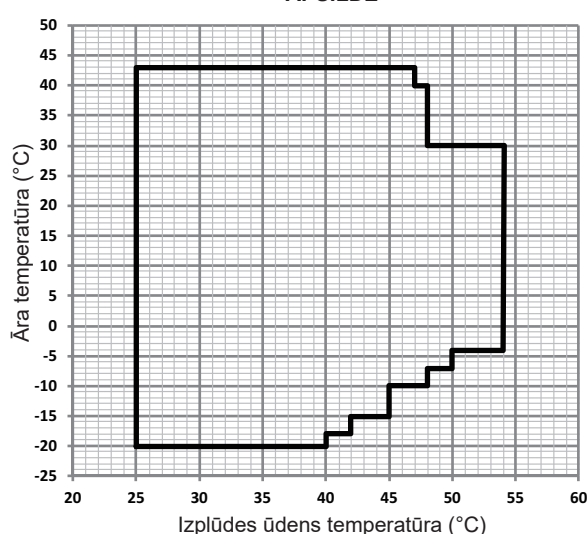
1-2-2. attēls. Apsildes darba diapazons
