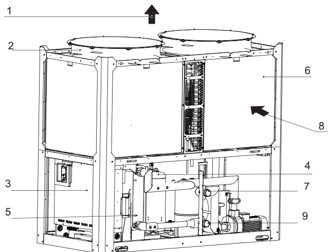
8-1. attēls. Modeļa KEM-75 DRS5 KH galvenās daļas (Attēls sniegts, tikai lai parādītu galveno daļu aptuvenu izvietojumu.)
