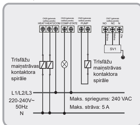
8-20. attēls. Ūdens sūkņa, cauruļu papildu sildītāja un kompresora stāvokļa maiņstrāvas indikatora elektroinstalācija (tikai modeļiem KEM-90 DRS5 KH un KEM-180 DRS5 KH)
