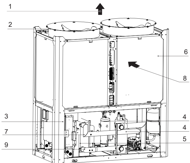
8-3. attēls. Modeļa KEM-140 DRS5 KH galvenās daļas (Attēls sniegts, tikai lai parādītu galveno daļu aptuvenu izvietojumu.)
