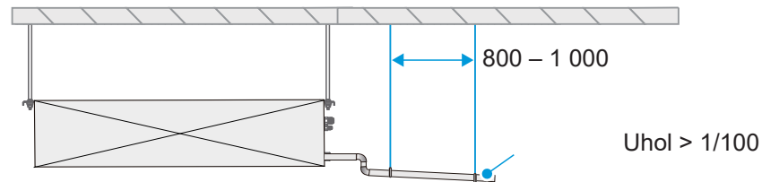
Spôsob pripojenia odtokového potrubia pre samostatnú jednotku
