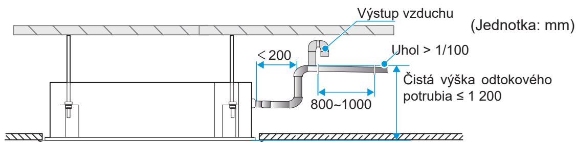
Spôsob pripojenia odtokového potrubia pre samostatnú jednotku
