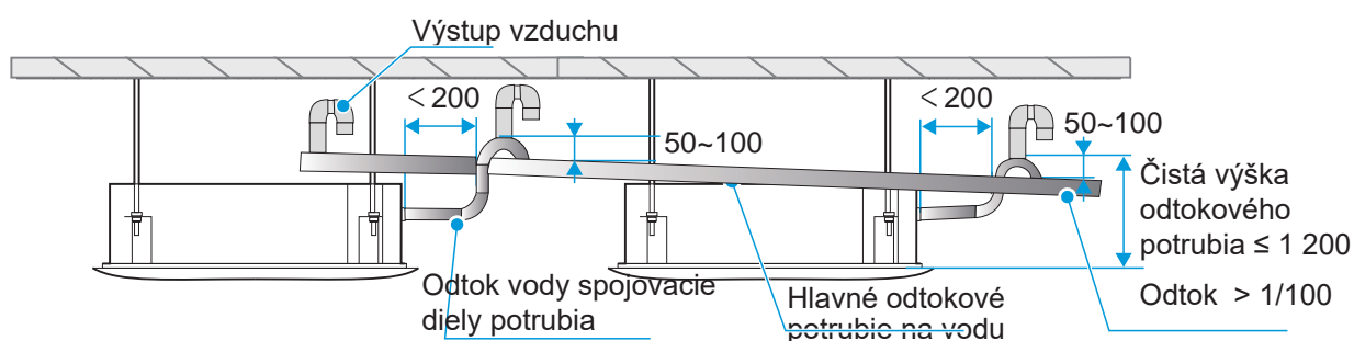
Odtokové potrubia z viacerých jednotiek sú napojené na hlavné odtokové potrubie, ktoré sa vypúšťa cez odpadové potrubie.
