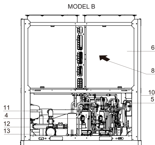
Afb. 8-4 Hoofdonderdelen van de KEM-180 DRS5 KH (De afbeelding wordt alleen gebruikt om de relatieve positie van de belangrijkste componenten weer te geven)
