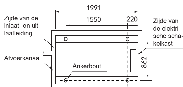
Afb. 6-6 Boven-aanzicht van het schema van de installatieafmetingen van KEM-75 DRS5 KH
