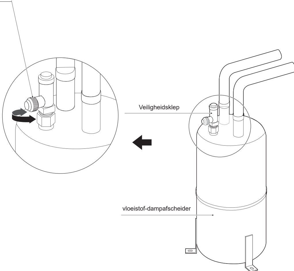
Fig.11-1 Vervanging van de veiligheidsklep
