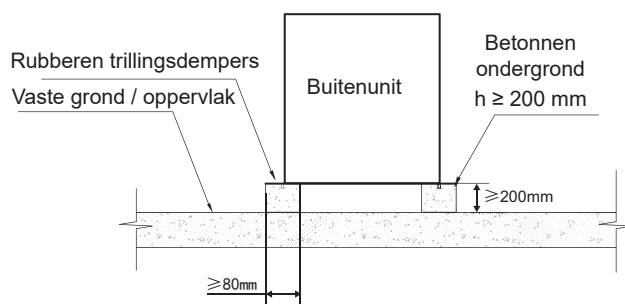
Afb. 6-5 Vooraanzicht van de basisstructuur
