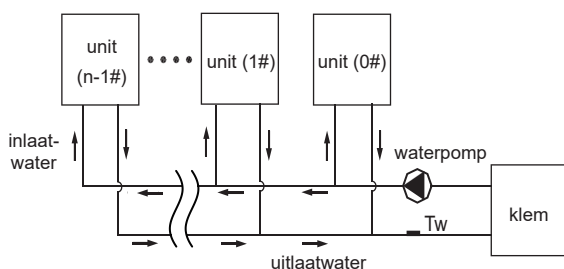
Afb. 8-33 Installatie van een enkele waterpomp
