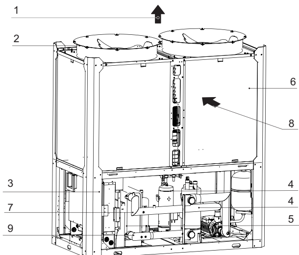
Afb. 8-3 Hoofdonderdelen van de KEM-140 DRS5 KH (De afbeelding wordt alleen gebruikt om de relatieve positie van de belangrijkste componenten weer te geven)
