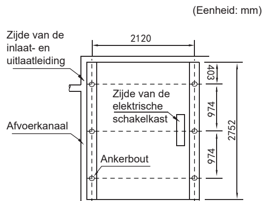
Afb. 6-8 Boven-aanzicht van het schema van de installatieafmetingen van KEM-180 DRS5 KH
