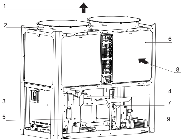
Afb. 8-1 Hoofdonderdelen van de KEM-75 DRS5 KH (De afbeelding wordt alleen gebruikt om de relatieve positie van de belangrijkste componenten weer te geven)
