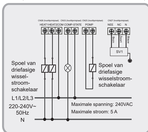
Afb. 8-20 Bedrading van de waterpomp en bijverwarming van de leidingen en ac-lampje van de status van de compressor (alleen voor KEM90 DRS5 KH en KEM-180 DRS5 KH)
