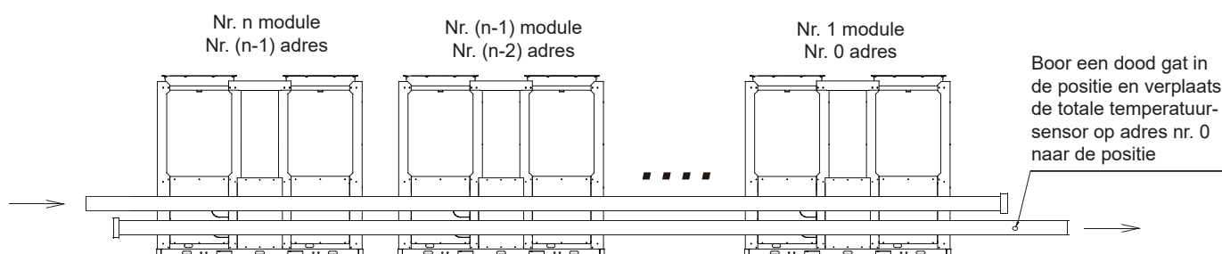
Afb. 8-32 Installatie van multimodulair systeem (niet meer dan 8 modules) KEM-180 DRS5 KH
