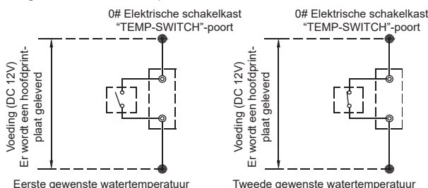
Afb. 8-22 Bedrading van "TEMP-SWITCH" zwakke elektrische poort
