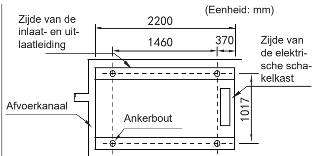
Afb. 6-7 Boven-aanzicht van het schema van de installatieafmetingen van KEM-90 DRS5 KH&MC-SU140M - RN8L-B
