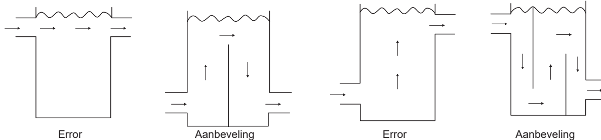
Afb. 8-26 Ontwerp van de opslagtank
