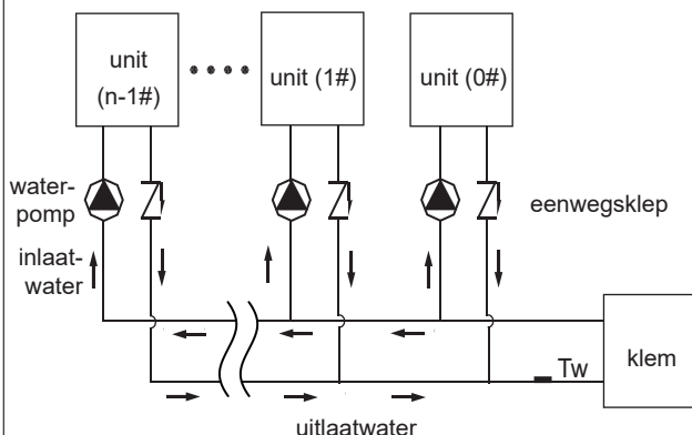
Afb. 8-34 Installatie van meerdere waterpompen
