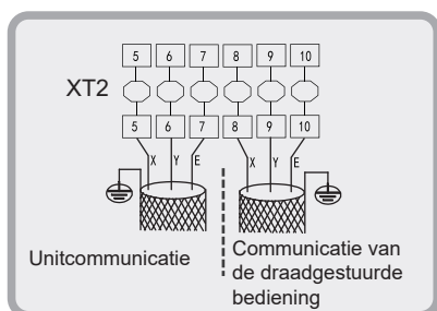
Afb. 8-18 Bedrading van de communicatie tussen unit en draadgestuurde bediening
