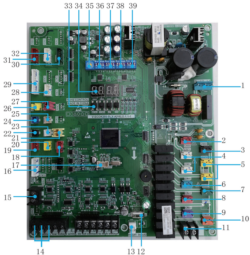
Afb. 8-9 hoofdprintplaat van de KEM-75 DRS5 KH en de KEM-140 DRS5 KH
