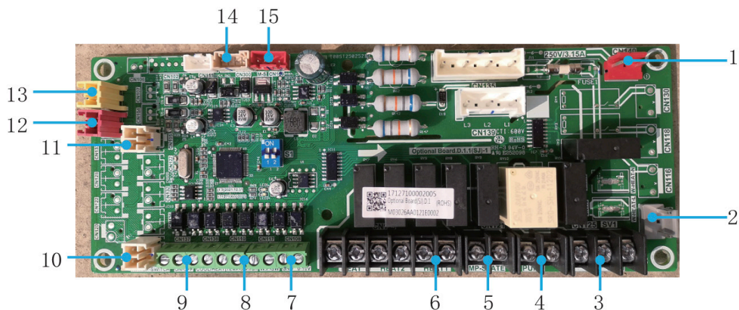
Afb. 8-10 Slavekaart van de MC-SU75-RN8L-B en MC-SU140-RN8L-B
