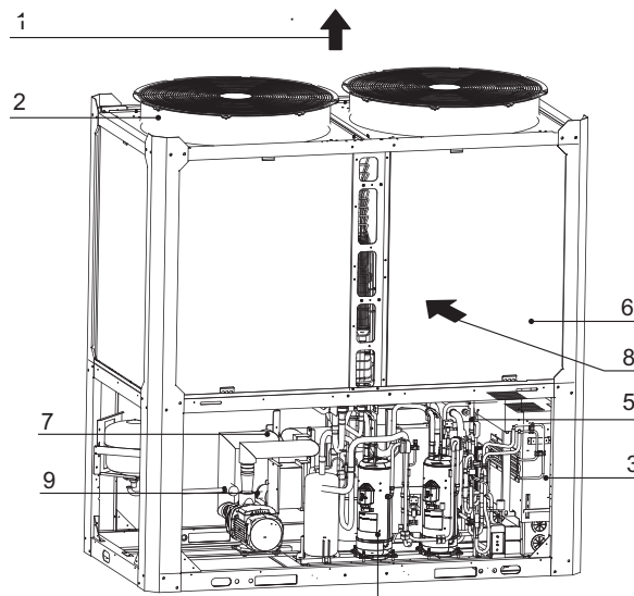
Afb. 8-2 Hoofdonderdelen van de MC SU90M-RN8L-B (De afbeelding wordt alleen gebruikt om de relatieve positie van de belangrijkste componenten weer te geven)
