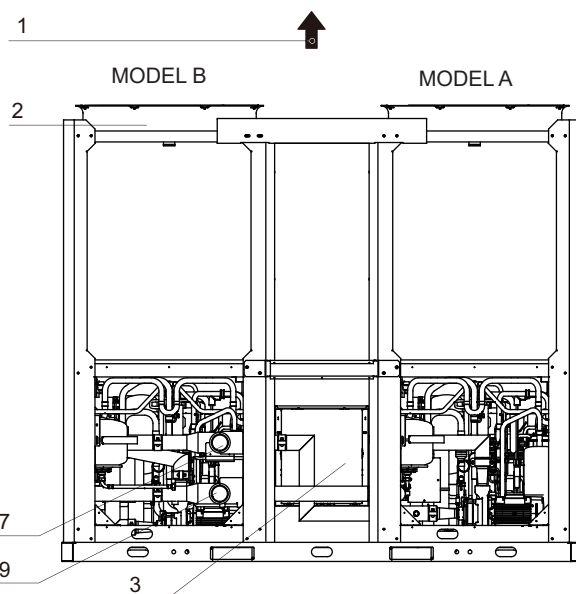
Afb. 8-4 Hoofdonderdelen van de KEM-180 DRS5 KH (De afbeelding wordt alleen gebruikt om de relatieve positie van de belangrijkste componenten weer te geven)
