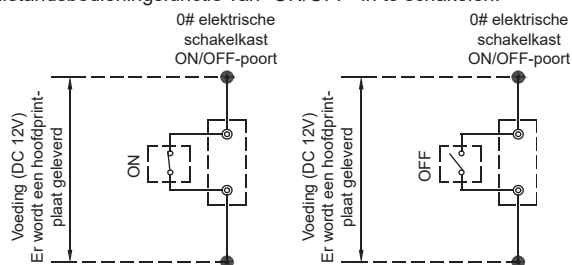
Afb. 8-21-1 Bedrading van "ON/OFF" zwakke elektrische poort
