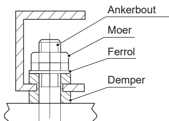
Afb. 6-9 Installatie van de demper
