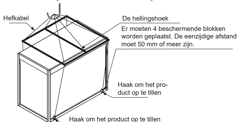
Afb. 3-1 Hissen van de unit
