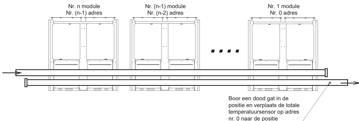
Afb. 8-31 Installatie van multimodulair systeem (niet meer dan 16 modules)
