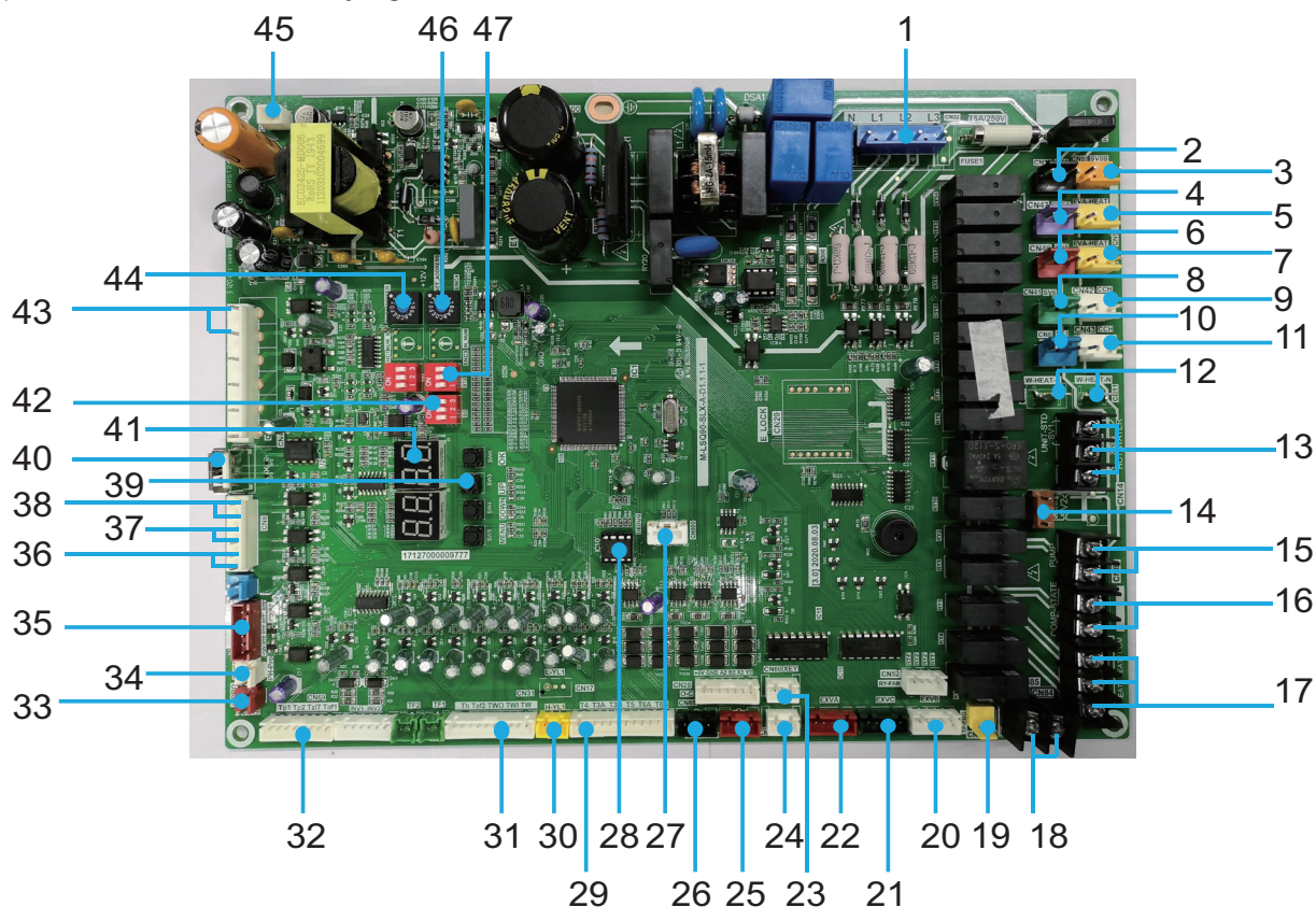
Afb. 8-11 Hoofdprintplaat van de KEM-90 DRS5 KH en de KEM-180 DRS5 KH
