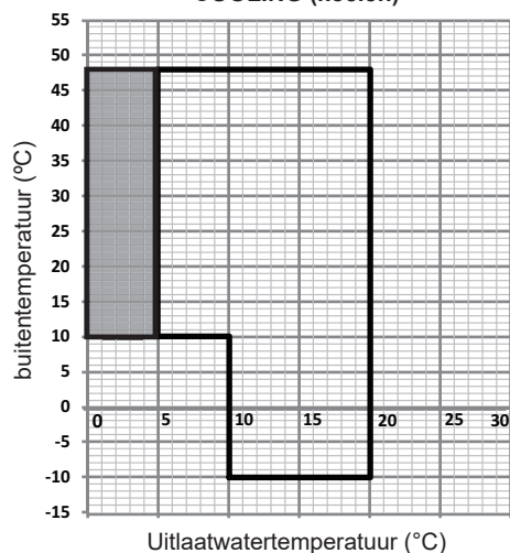
Afb. 1-1-1 Koelbereik
