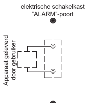
Afb. 8-23 Bedrading van "ALARM"-poort
