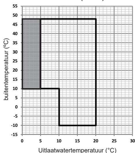
Afb. 1-1-2 Koelbereik
