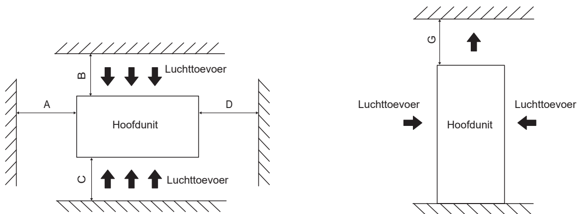
Afb. 6-3 Installatie van één unit
