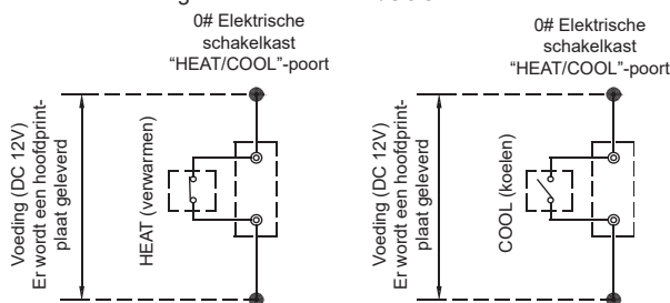
Afb. 8-21-2 Bedrading van "HEAT/COOL" zwakke elektrische poort
