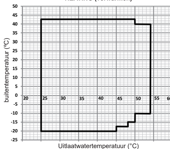
Afb. 1-1-2 Verwarmingsbereik
