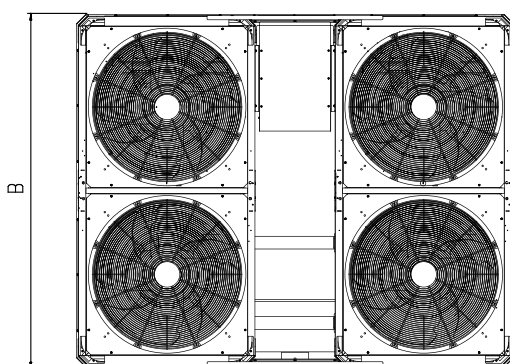
Bovenaanzicht
