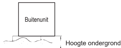
Afb. 6-11 Basishoogte voor sneeuwpreventie
