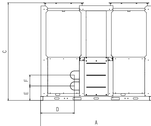
Vooraanzicht
