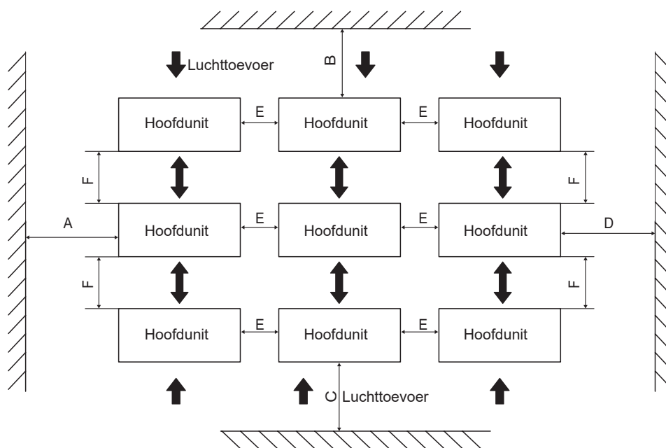
Afb. 6-4 Installatie van meerdere units
