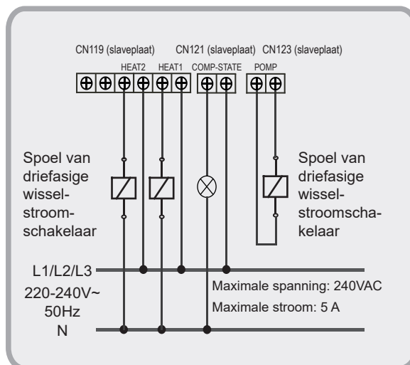
Afb. 8-19 Bedrading van de waterpomp en bijverwarming van de leidingen en ac-lampje van de status van de compressor (alleen voor KEM75 DRS5 KH en KEM-140 DRS5 KH)
