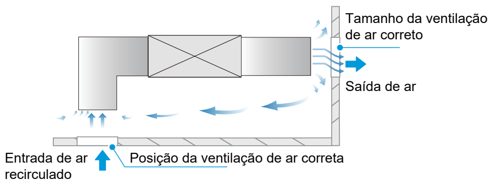
Tamanho e posição da ventilação de ar corretos
