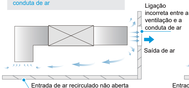
Ligação incorreta entre a ventilação e a conduta de ar
