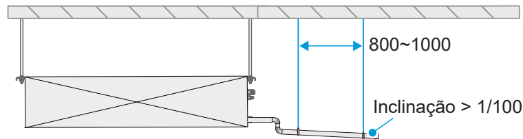
Método para ligar o tubo de drenagem para uma unidade individual
