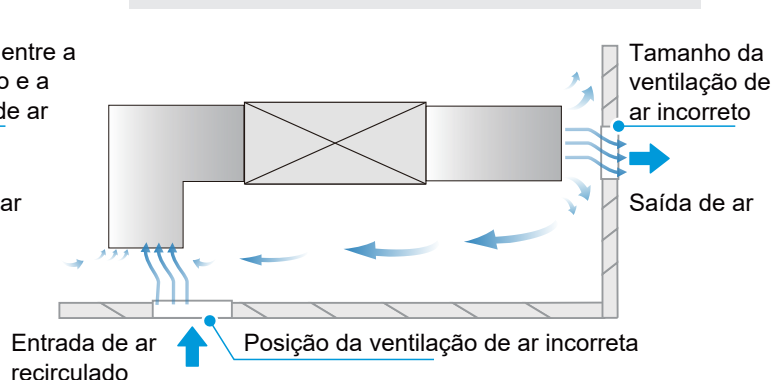
Tamanho e posição da ventilação de ar incorretos
