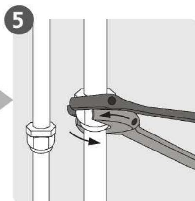
Podłącz przewody rurowe
