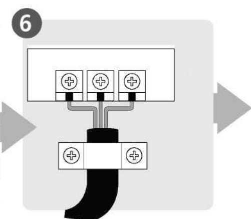
Podłącz przewody (nie dotyczy niektórych lokalizacji w Ameryce Północnej)
