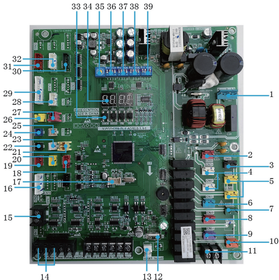
III. 8-5 Carte principale des modèles de 65 kW et 110 kW
