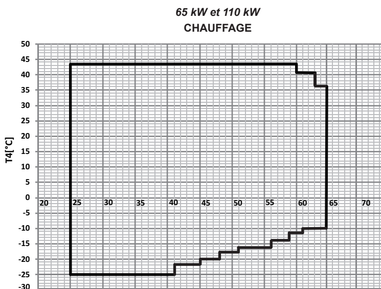
Two [°C] Température de sortie d'eau (°C)
