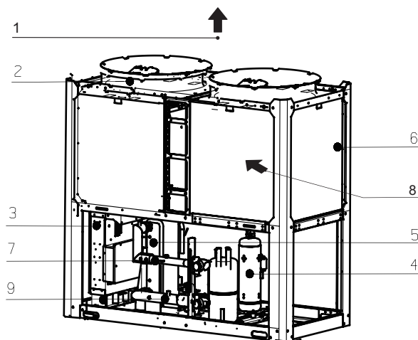
III. 8-1 Pièces principales de 65 kW
