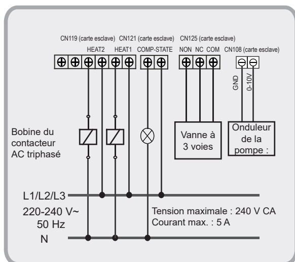
III. 8-11 Câblage du chauffage auxiliaire de conduites et Voyant CA de l'état du compresseur (65 kW et 110 kW)
