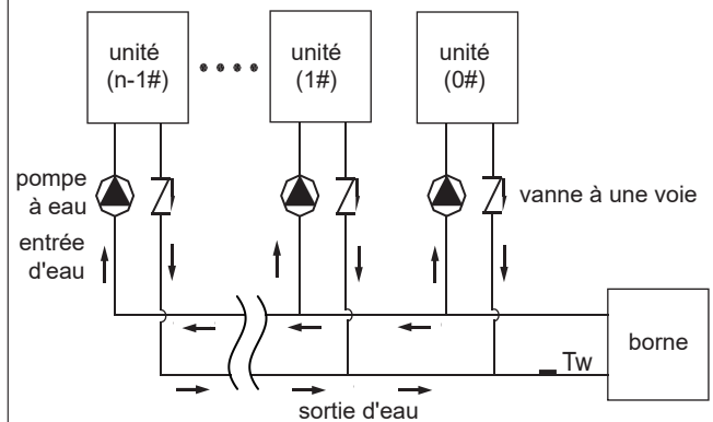
III.8-24 Installation de plusieurs pompes à eau
