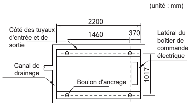
III. 6-6 Vue du dessus du schéma des dimensions de l'installation de 110 kW
