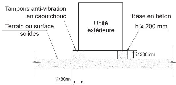
III.6 -4 Vue de face de la structure de base
