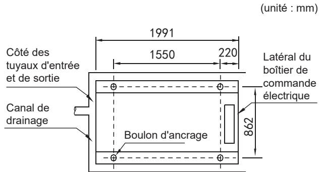
III. 6-5 Vue du dessus du schéma des dimensions de l'installation de 65 kW
