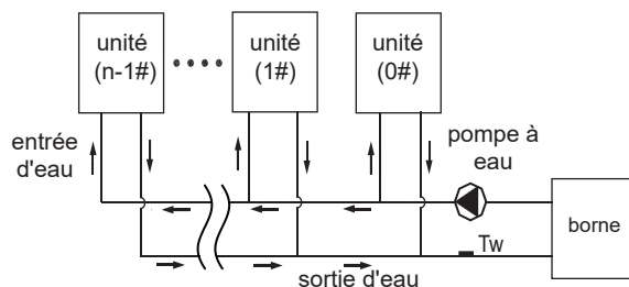
III.8-23 Installation d'une ou plusieurs pompes à eau
