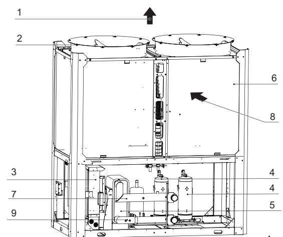
III. 8-2 Pièces principales de 110 kW
