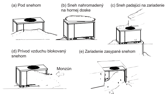
Obr. 6 – 9 Typy problémov spôsobené snehom
