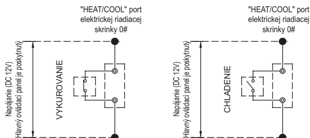
Obr. 8 – 15 Zapojenie slaboprúdového portu „HEAT/COOL“
