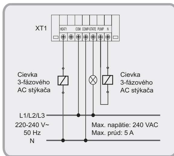
Obr. 8 – 13 Zapojenie vodného čerpadla a prídavného ohrievača potrubia a striedavého svetla stavu kompresora
