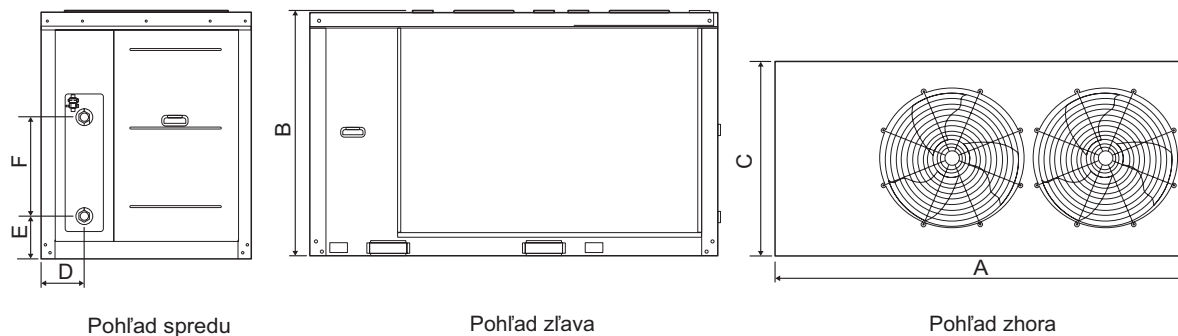
Obr. 6 – 2 Náčrt rozmerov KEM-60 DRS4 KH
