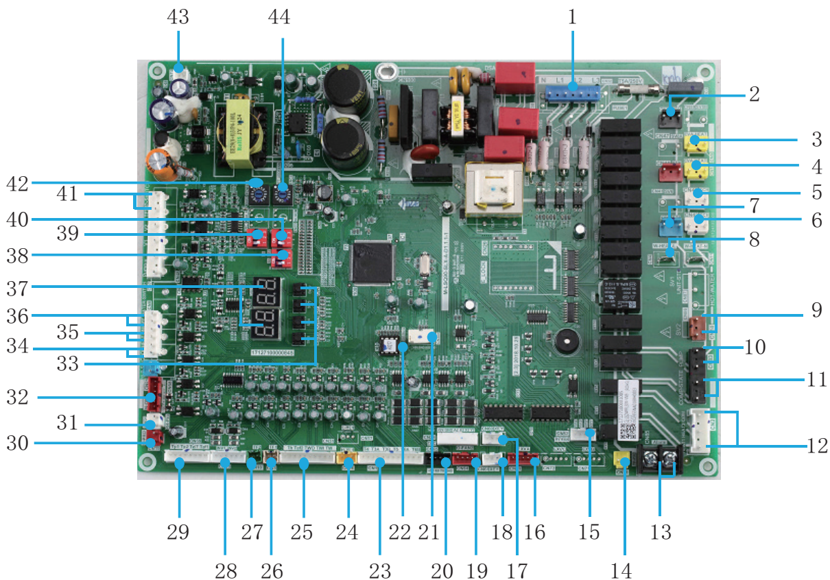
Obr. 8 – 7 Hlavná DPS KEM-30 DRS4 KH a KEM-60 DRS4 KH
