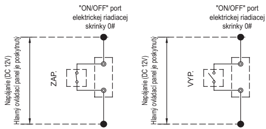
Obr. 8 – 14 Zapojenie slaboprúdového portu "ON/OFF"
