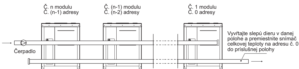
Obr.8-24 Inštalácia viacmodulového zariadenia (maximálne 16 modulov)
