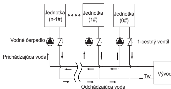
Obr.8-26 Inštalácia viacerých vodných čerpadiel
