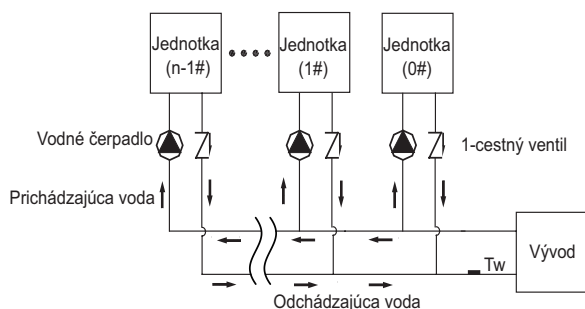
Obr.8-25 Inštalácia jedného vodného čerpadla
