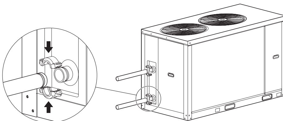
Obr.8-21 spôsob pripojenia potrubia KEM-60 DRS4 KH
