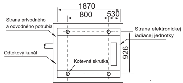
Obr. 6 – 6 Pohľad zhora na schému montážnych rozmerov KEM-30 DRS4 KH
