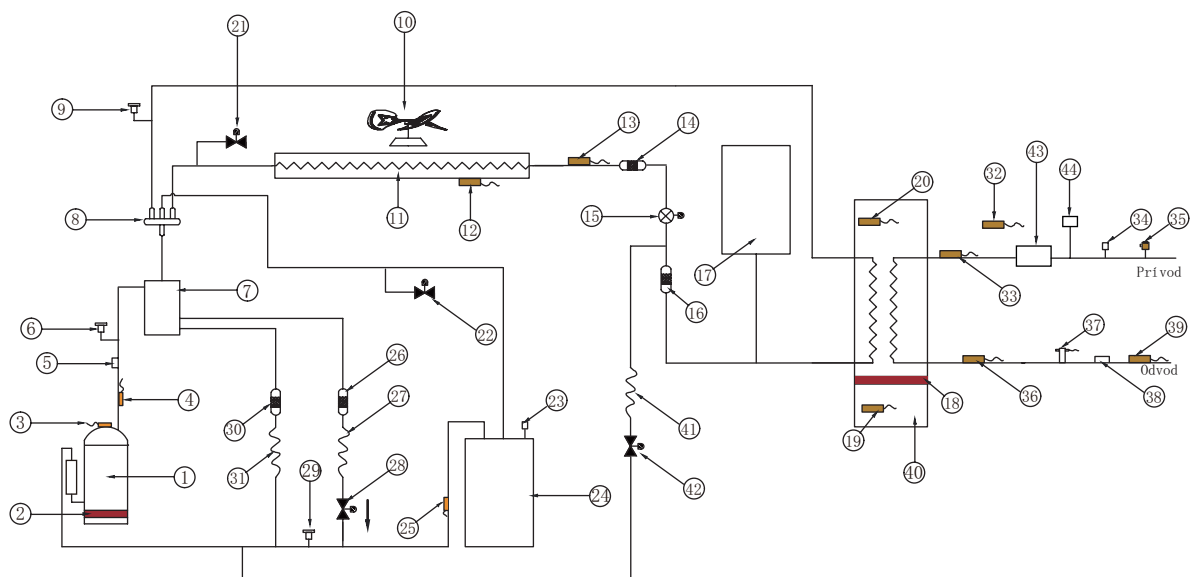
Obr. 8 – 5 Funkčná schéma KEM-30 DRS4 KH
