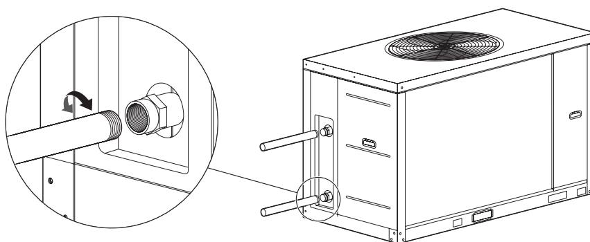
Obr.8-20 spôsob pripojenia potrubia KEM-30 DRS4 KH
