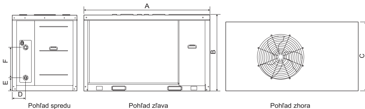
Obr. 6 – 1 Náčrt rozmerov KEM-30 DRS4 KH
