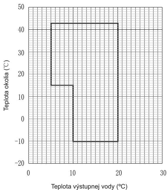
Obr. 1-1 Preádzkový rozsah chladenia KEM-30 DRS4 KH a KEM-60 DRS4 KH
