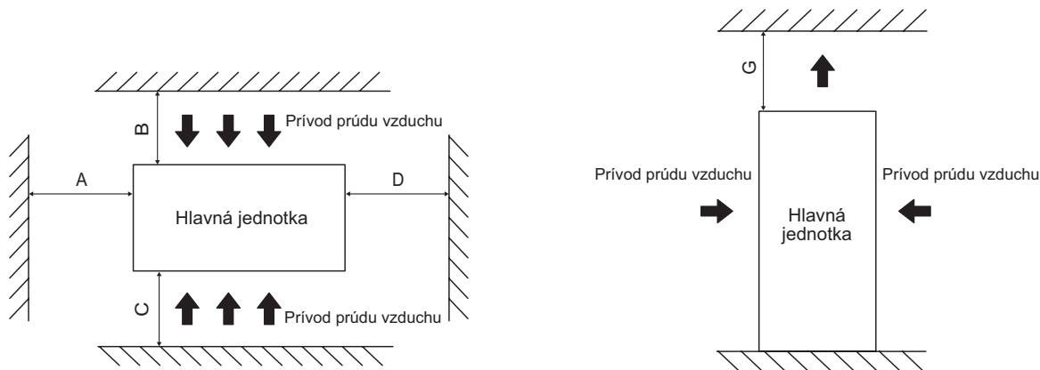
Obr. 6 – 3 inštalácia jednej jednotky
