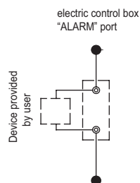
Obr. 8 – 16 Zapojenie portu „ALARM“
