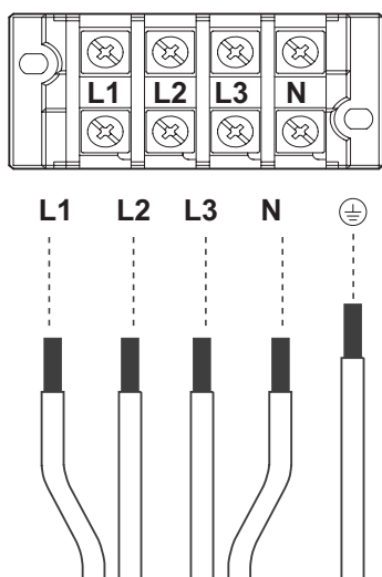
Obr. 8 – 11 Požiadavky na pripojenie
