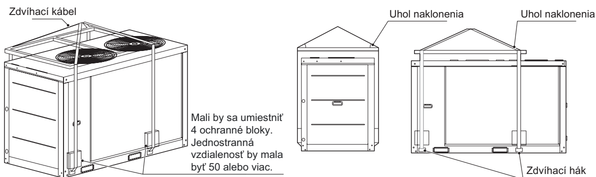
Obr. 3 – 1 zdvíhanie jednotky
