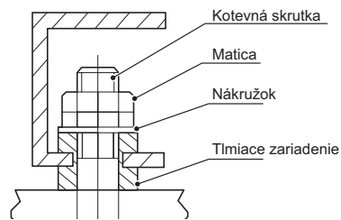
Obr. 6 – 8 Inštalácia tlmiča
