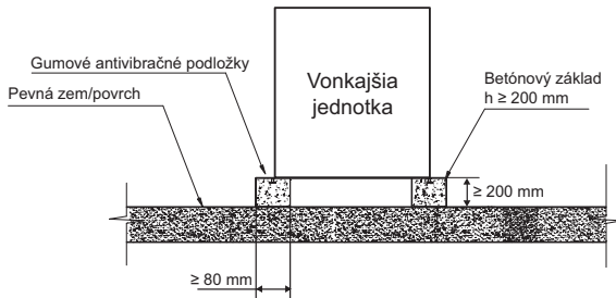
Obr. 6 – 5 Pohľad spredu na základnú konštrukciu
