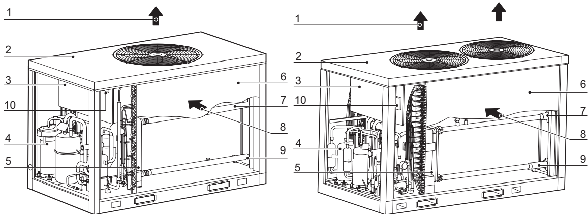
Obr. 8 – 1 Hlavné diely KEM-30 DRS4 KH Obr. 8 – 2 Hlavné diely KEM-60 DRS4 KH
