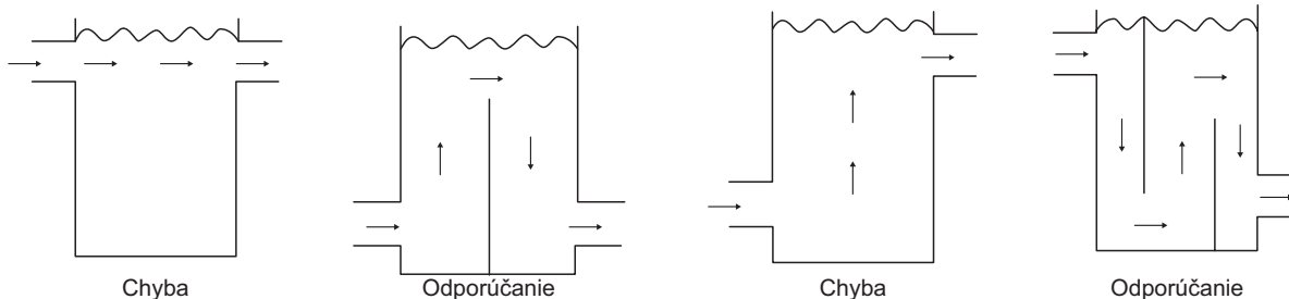
Obr.8-22 Konštrukcia akumuláčnej nádrže
