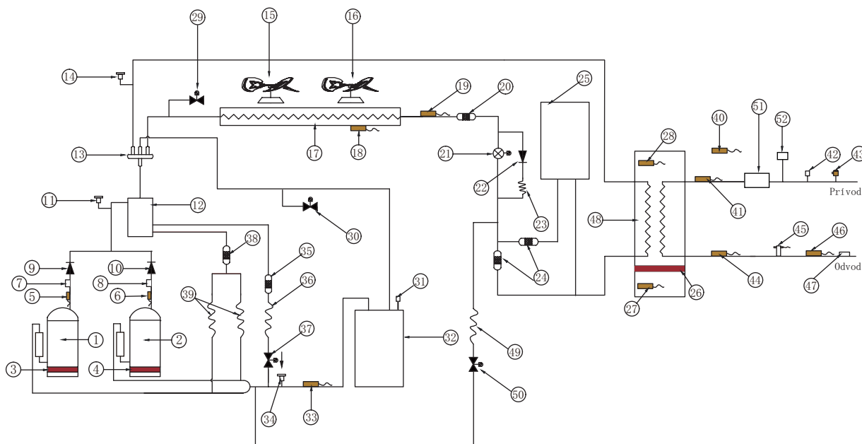
Obr. 8 – 6 Funkčná schéma KEM-60 DRS4 KH
