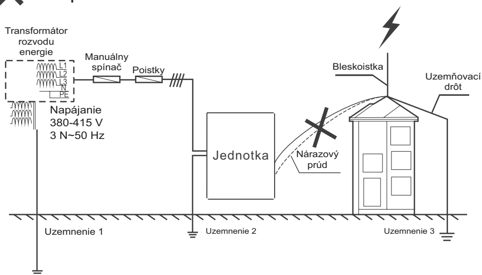
Obr. 8 – 10 Požiadavky na kabeláž napájania
