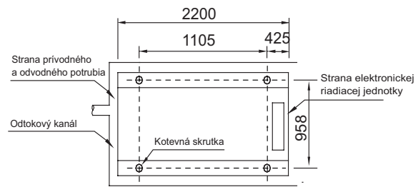
Obr. 6 – 7 Pohľad zhora na schému montážnych rozmerov KEM-60 DRS4 KH
