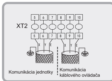
Obr. 8 – 12 Zapojenie komunikácie jednotky a komunikácie káblového ovládača
