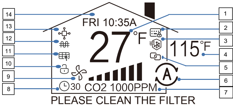
Sch. 25 Interface principale de l'affichage (Pour VRC)
