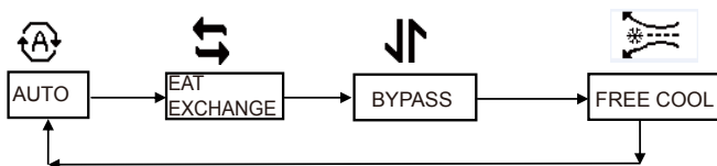
Sch. 27 Réglage de mode
