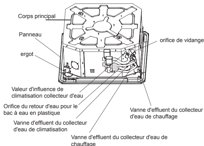
Cassette à quatre voies (compacte)
