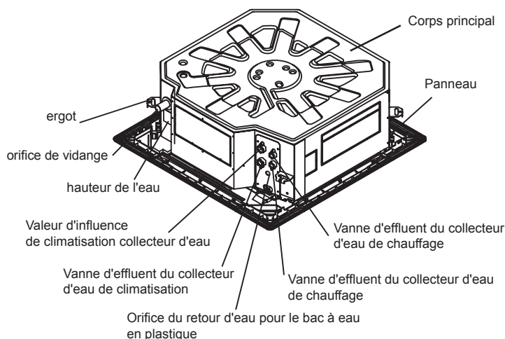
Cassette à quatre voies
