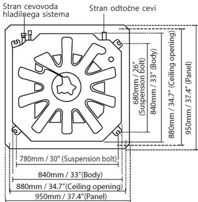
18-48K velikost odprtine v stropu za Super-Slim modele
