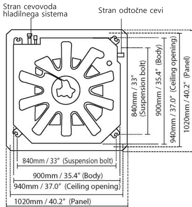
60K velikost odprtine v stropu za Super-Slim modele
