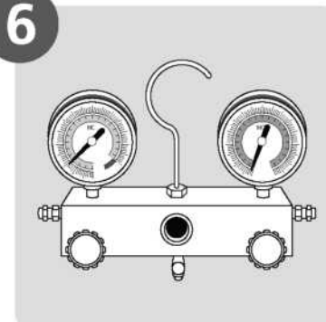
Evacue o sistema de refrigeração
