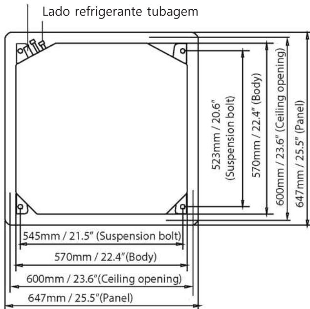
Tamanho do orifício do teto dos modelos compactos
