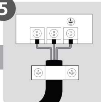
Ligue os fios
