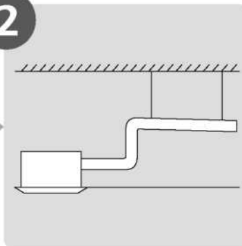
Instalação da tubo de drenagem
