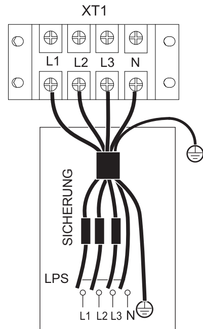
INNENGERÄTE-SPANNUNGS VERSORGUNG 3-phasiger 9kW-Reserveveizer Angepasst
