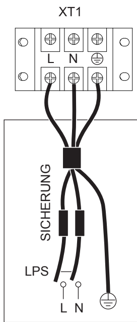
INNENGERÄTE-SPANNUNGS VERSORGUNG 1-phasiger 3kW-Reserveveizer Standard
