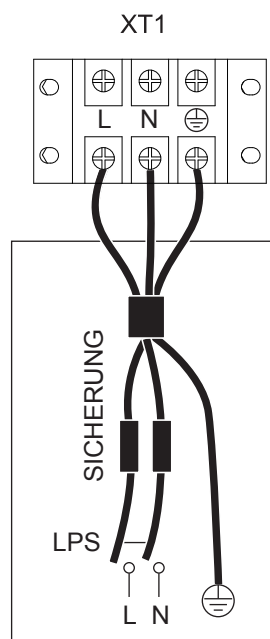
INNENGERÄTE-SPANNUNGS VERSORGUNG 1-phasiger 6kW-Reserveveizer Angepasst
