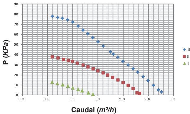
Caudal VS de la presión estática externa disponible (monofásica 10-16 kW + trifásica 12~16 kW)
