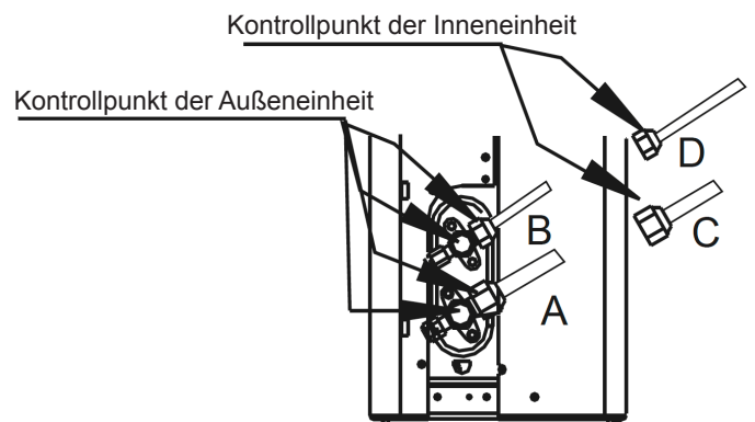
A: Niederdruck-Sperrventil B: Hochdruck-Sperrventil C & D: Muttern der Inneneinheit
